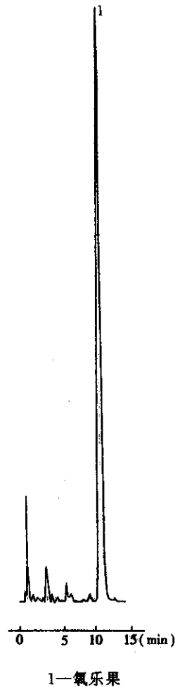
图1 氧乐果乳油高效液相色谱图
